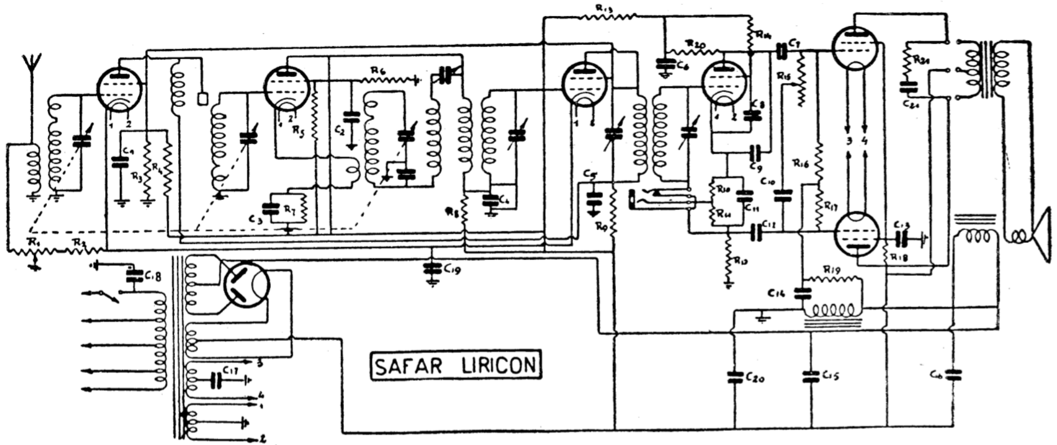
SAFAR RADIO. — Mod. Liricon. — Valvole: V1 = '35; V2 = '24; V3 = '35; V4 = '24; V5, V6 = '47; V7 = '80. MF: 175 kHz. — Produzione 1932.
